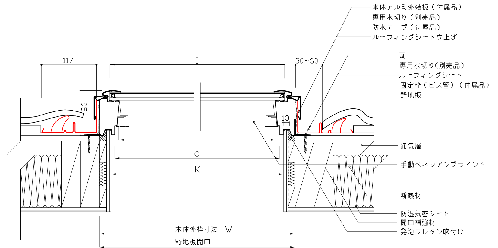
横断面図
